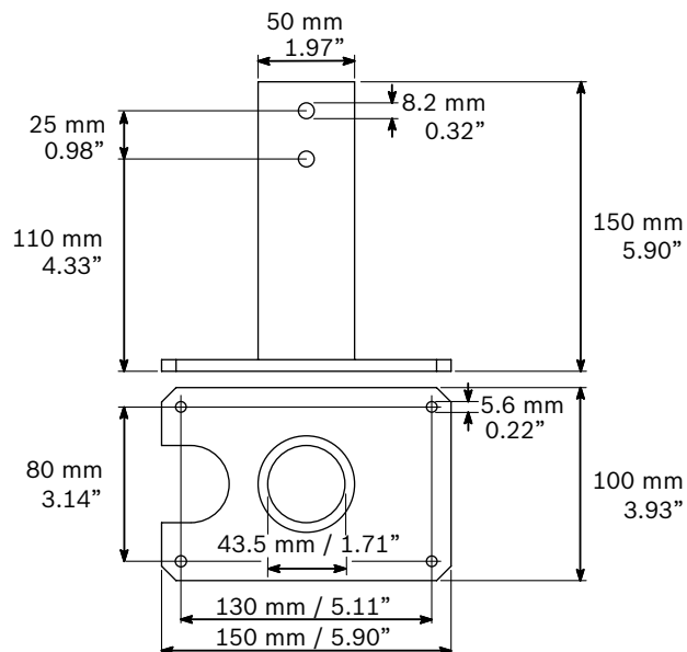
Dimensions LM1-MSB-1
