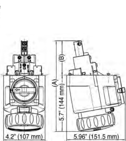
FLANGE RECEPTACLE 30A 3 POLE - 4 WIRE & 4 POLE - 5 WIRE 8571/25-...
