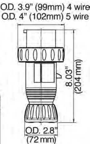
PLUG 30A 3 POLE - 4 WIRE & 4 POLE - 5 WIRE 8571/2-...
