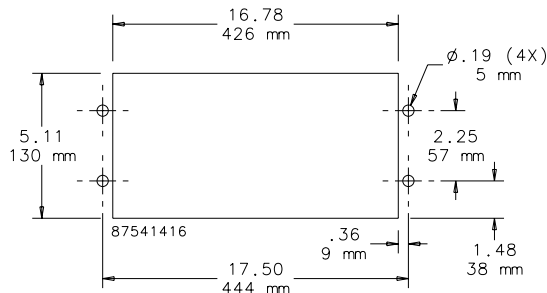
CUTOUT DIMENSIONS
