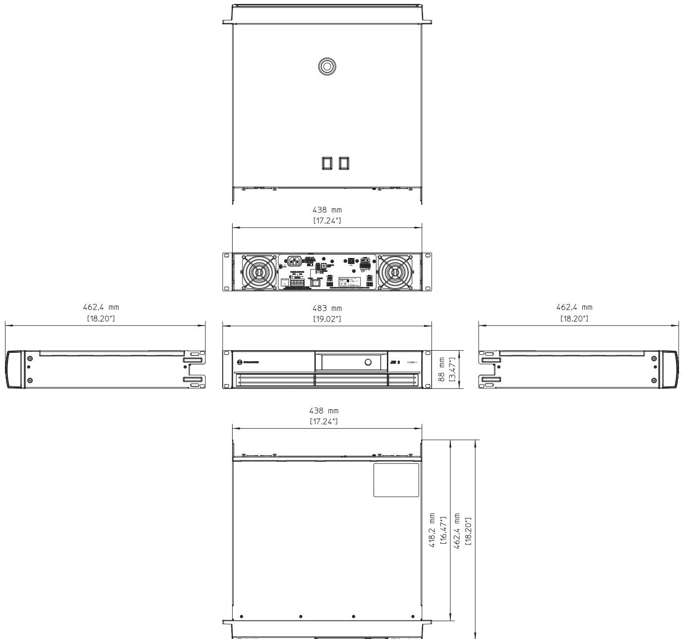
Dimensions
