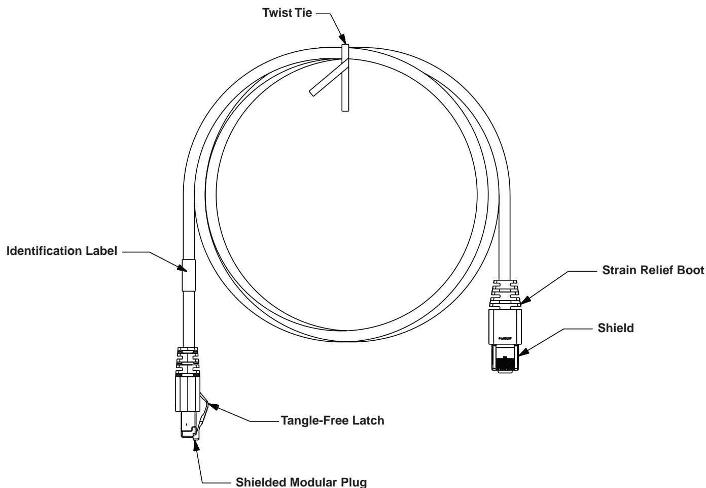
T568A Wiring Scheme
