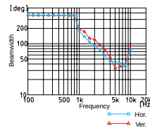
Beamwidth
