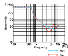
Beamwidth
