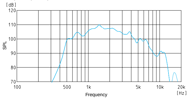
Beamwidth
