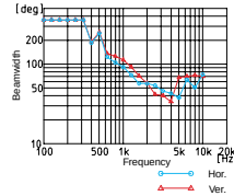
Beamwidth
