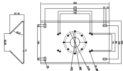
L3PTZPOLEMT Lineart
